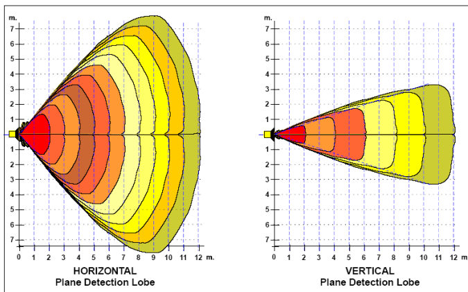
Horizontale en verticale detectieveld bij 12 meter uitvoering
