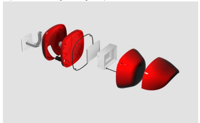
Opbouw behuizing met regenkap
